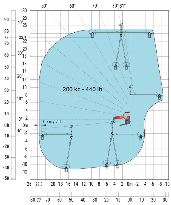
支腿完全打开 车身旋转 带 3D平台 正向/负向
