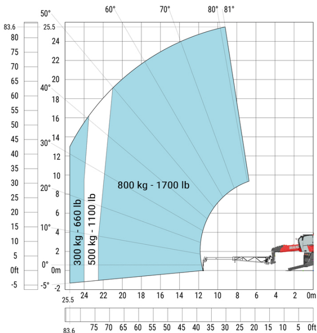
支腿打开 带有卷扬的可伸缩吊臂 公制
