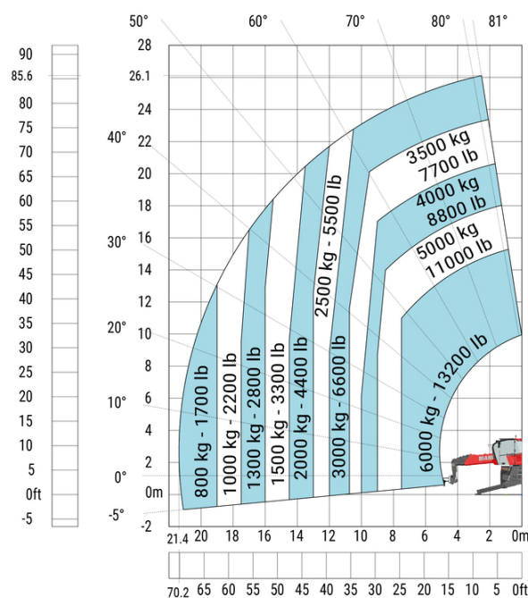
支腿打开 带 6000 kg 吊钩 公制
