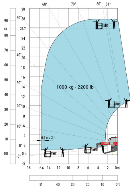
支腿完全打开 车身旋转 带 1000 kg工作平台
