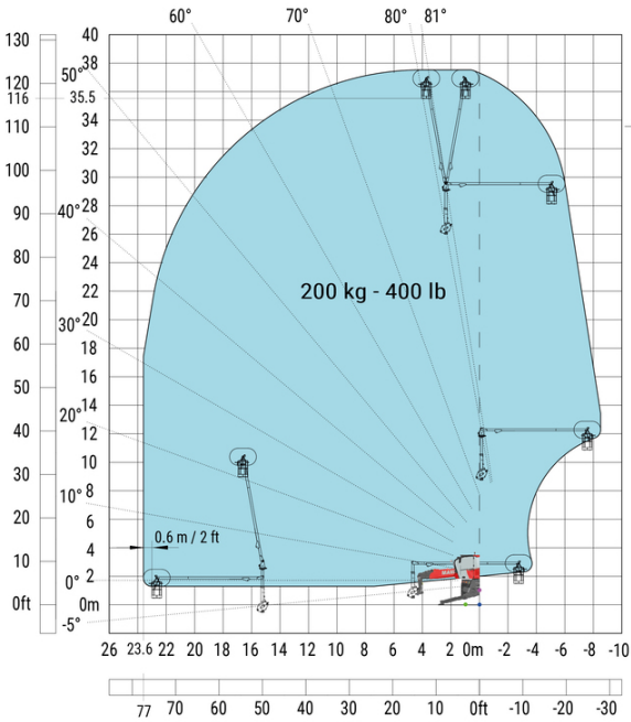
支腿完全打开 车身旋转 带 3D 平台 正向
