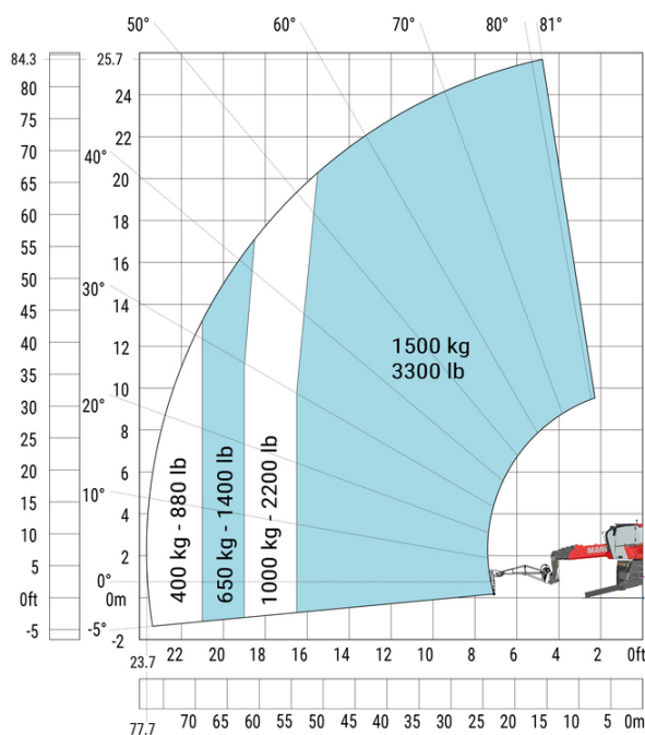
支腿打开 带 1500 kg 有卷扬的吊臂 公制
