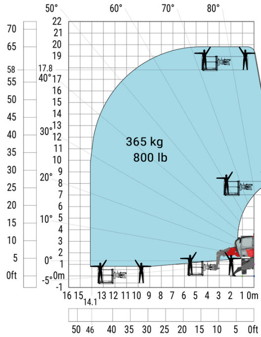
支腿完全打开 车身旋转 带 365 kg工作平台
