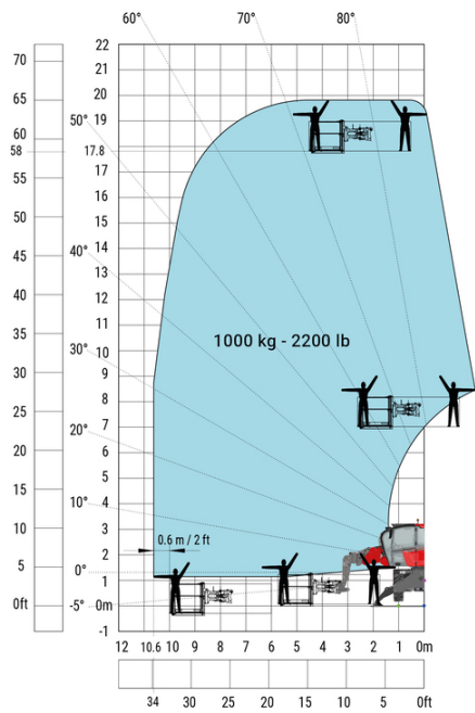
支腿完全打开 车身旋转 带 1000 kg工作平台
