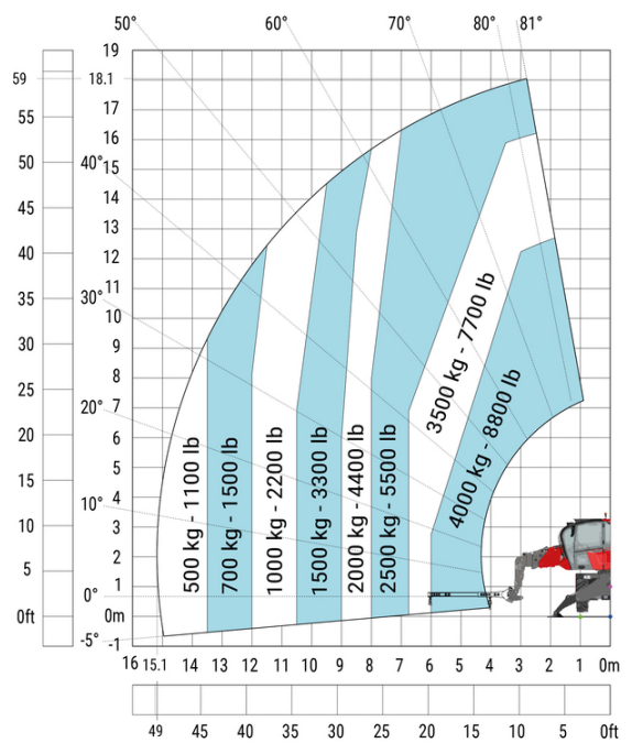
支腿打开 带 4000 kg 吊臂 公制
