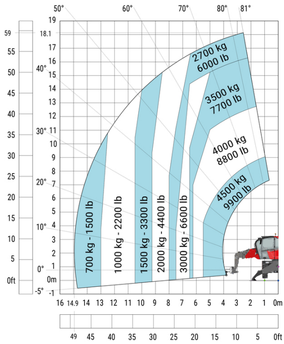
支腿打开 带 5000 kg 吊钩 公制
