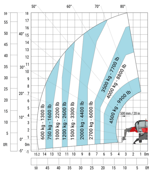
支腿完全打开 车身旋转 带货叉
