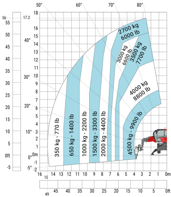
支腿完全打开 车身旋转 带 5000 kg卷扬机
