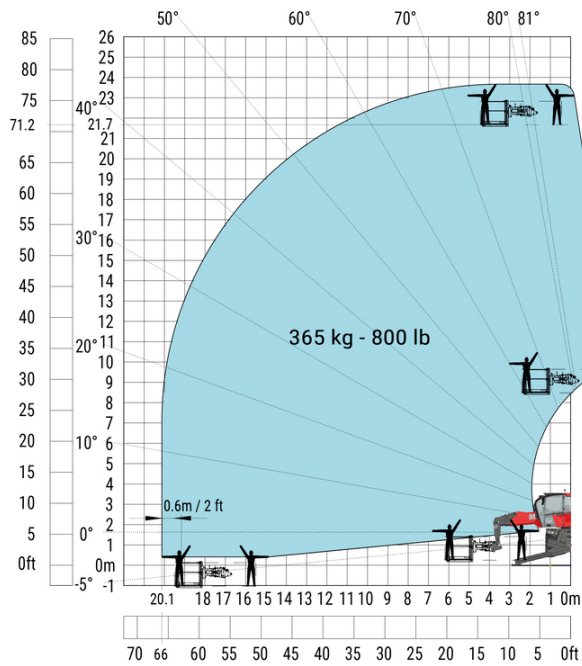
支腿完全打开 车身旋转 带 365 kg工作平台
