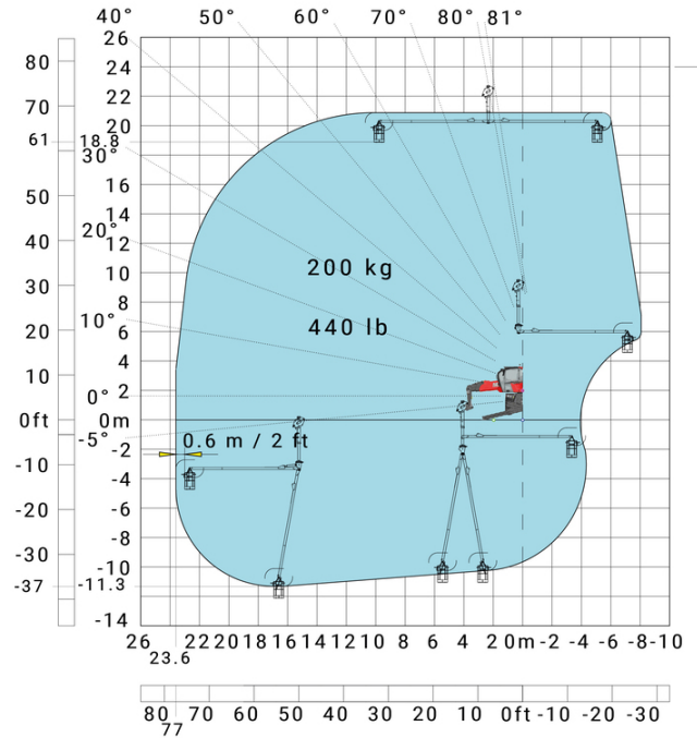
支腿完全打开 车身旋转 带 3D平台 正向/负向
