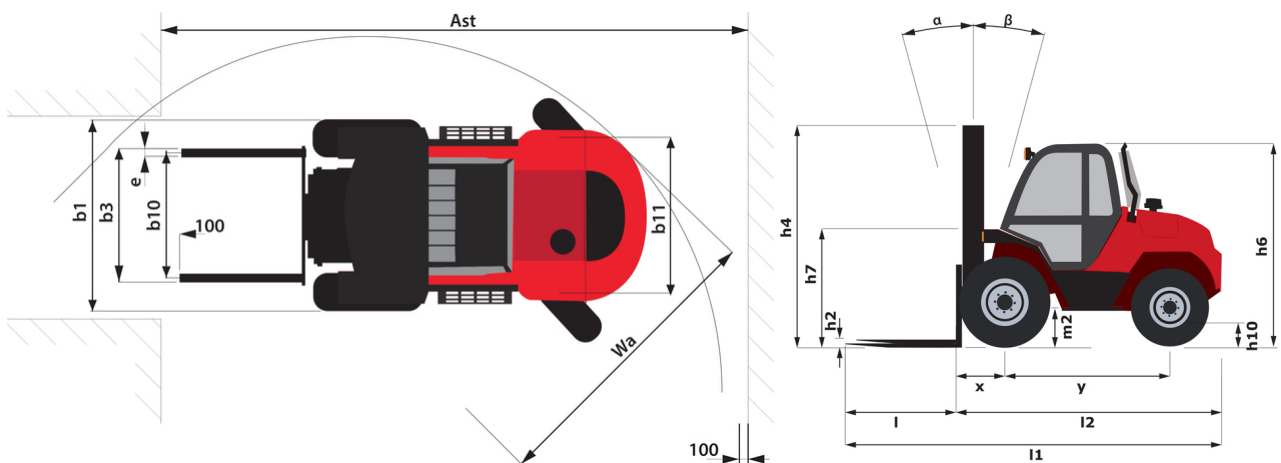
M-X 50-4 - 尺寸图
