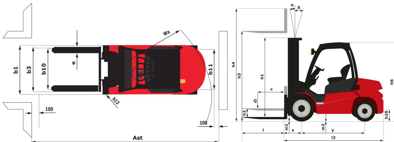
MI-X 35 G - 尺寸图
